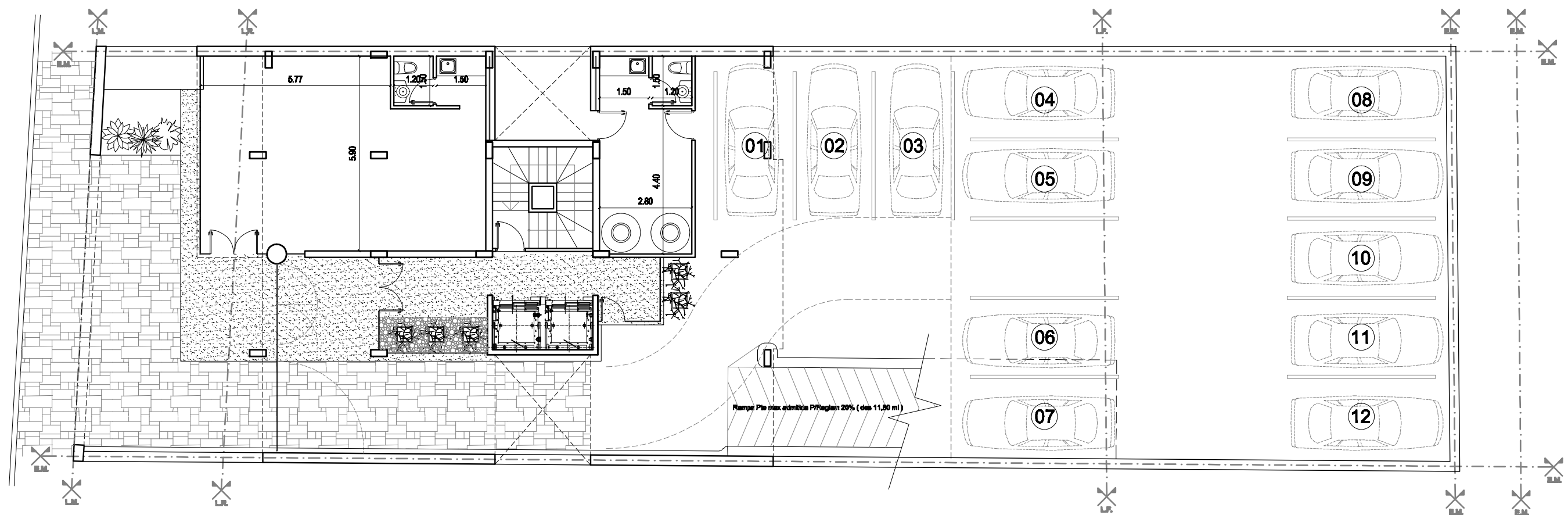
PLANTA BAJA
