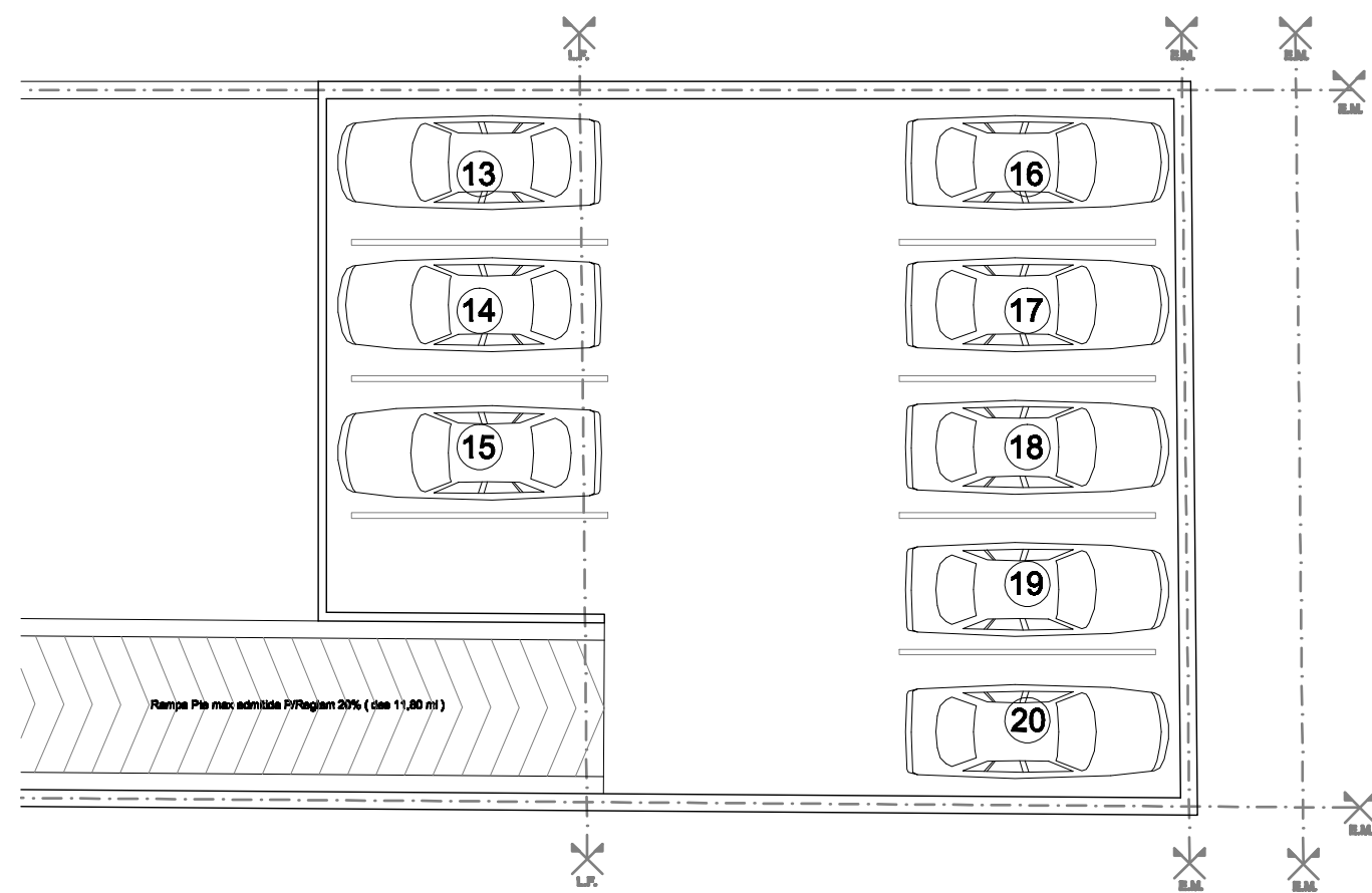
ENTREPISO COCHERAS
